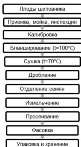
Рисунок 2 – Структурная схема получения порошка из семян шиповника
