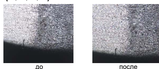
Рисунок 7 – Микроструктура испытания на МКК по методу АМУ, продолжительность кипячения – 8 часов
