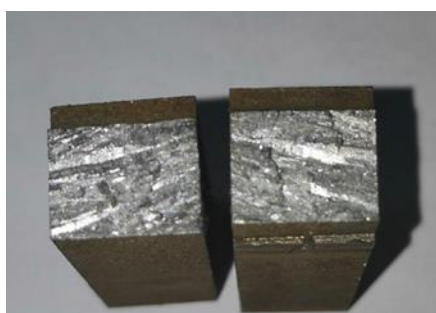
Рисунок 2 – Фото излома образца системы Al-Co-Cr-Fe-Mn после проведения испытания на ударную вязкость
